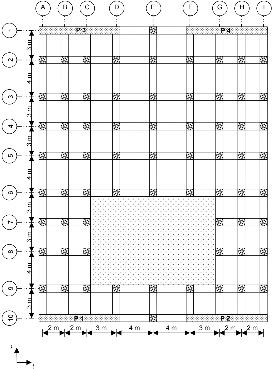
Şekil 5.21. Örnek 5.15'nin kat kalıp planı
