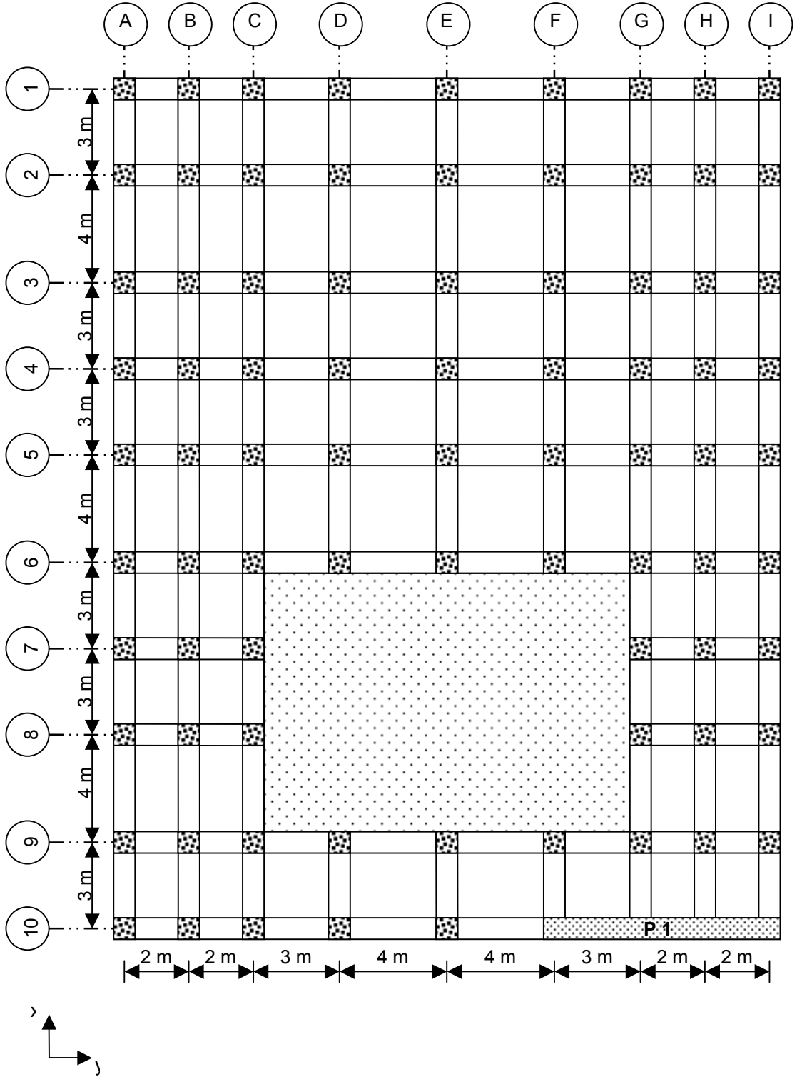
Şekil 5.15. Örnek 5.9'nin kat kalıp planı
