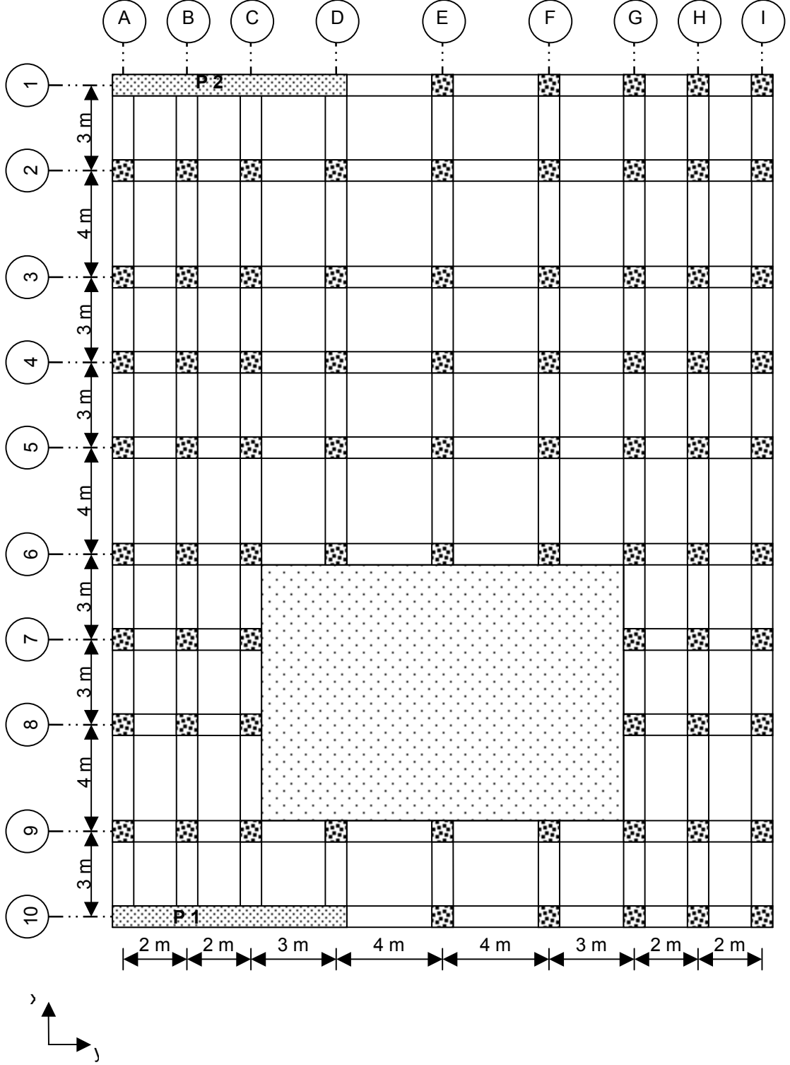
Şekil 5.17. Örnek 5.11'nin kat kalıp planı
