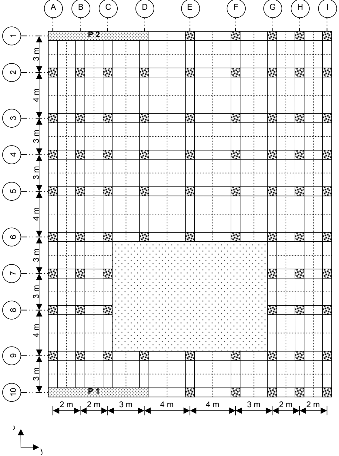
Şekil 5.18. Örnek 5.12'in kat kalıp planı
