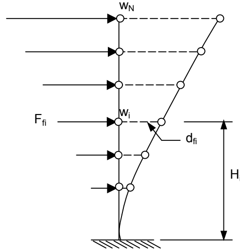
Şekil 4.1. Fiktif yükler ve yer değiştirmeler
